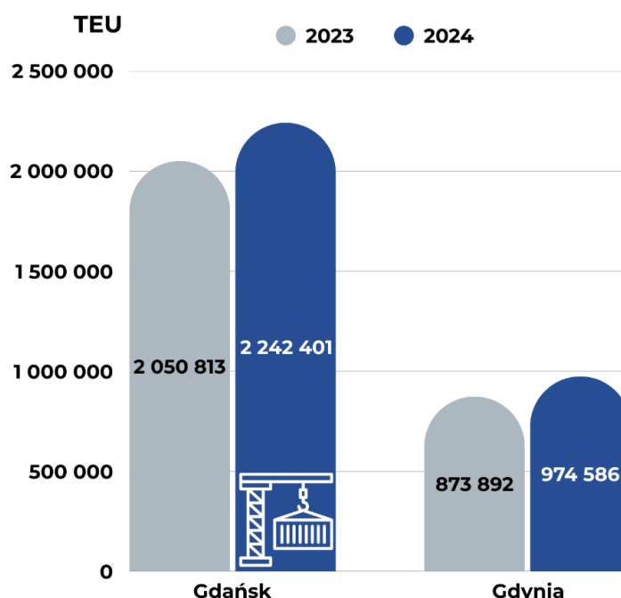
Ryc. 27. Przeładunki kontenerów
