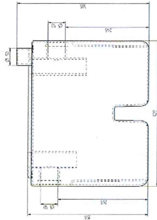
Rys. 4 Oddzielnik tłuszczu - widok z boku
