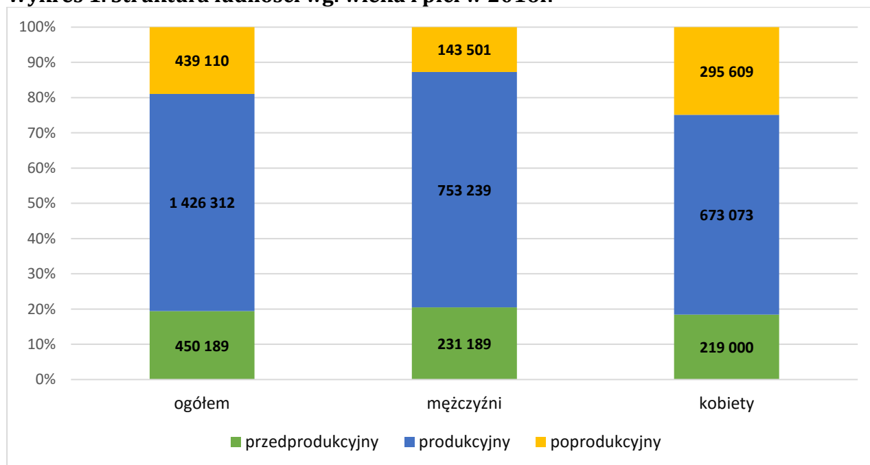
Wykres 1. Struktura ludności wg. wieku i płci w 2016r.
