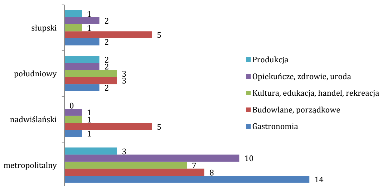
Wykres 6. Profile działalności spółdzielni socjalnych
