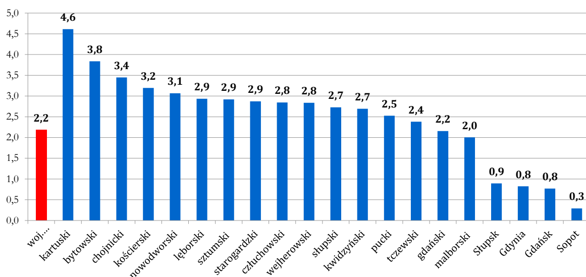
Wykres 2. Odsetek rodzin wielodzietnych w stosunku do rodzin z dziećmi w ogóle wg. powiatów
