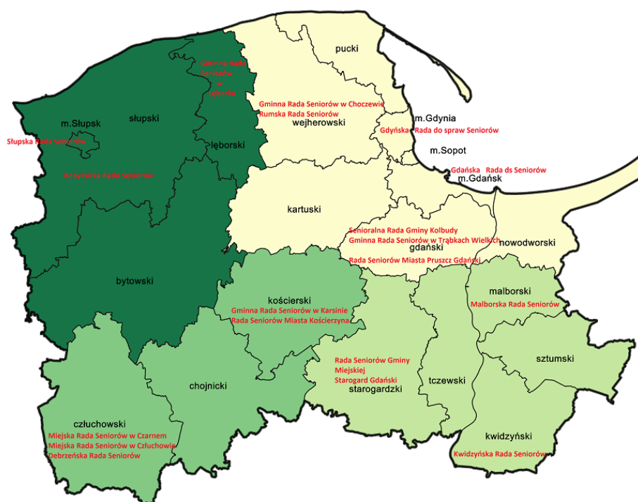
Mapa 2. Rady Seniorów w pomorskich subregionach.
