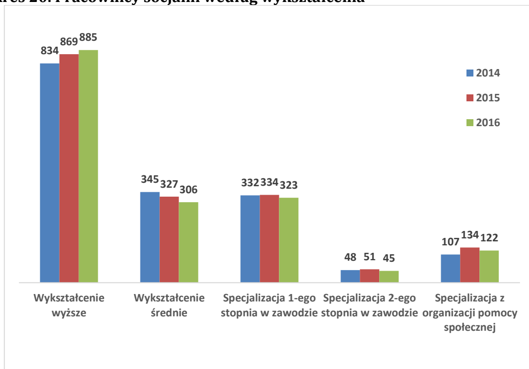
Wykres 20. Pracownicy socjalni według wykształcenia
