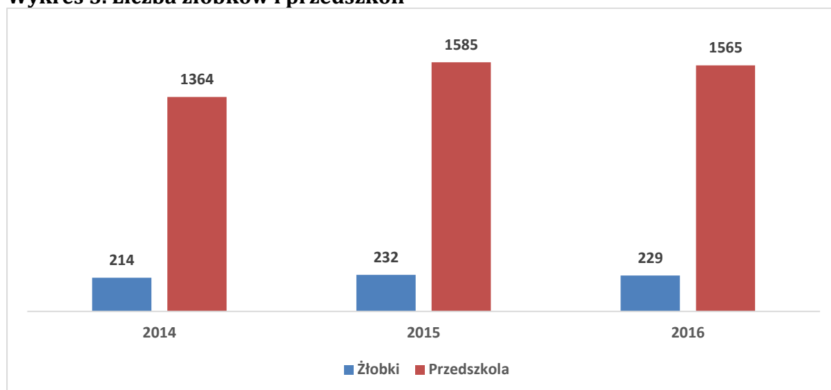
Wykres 5. Liczba żłobków i przedszkoli
