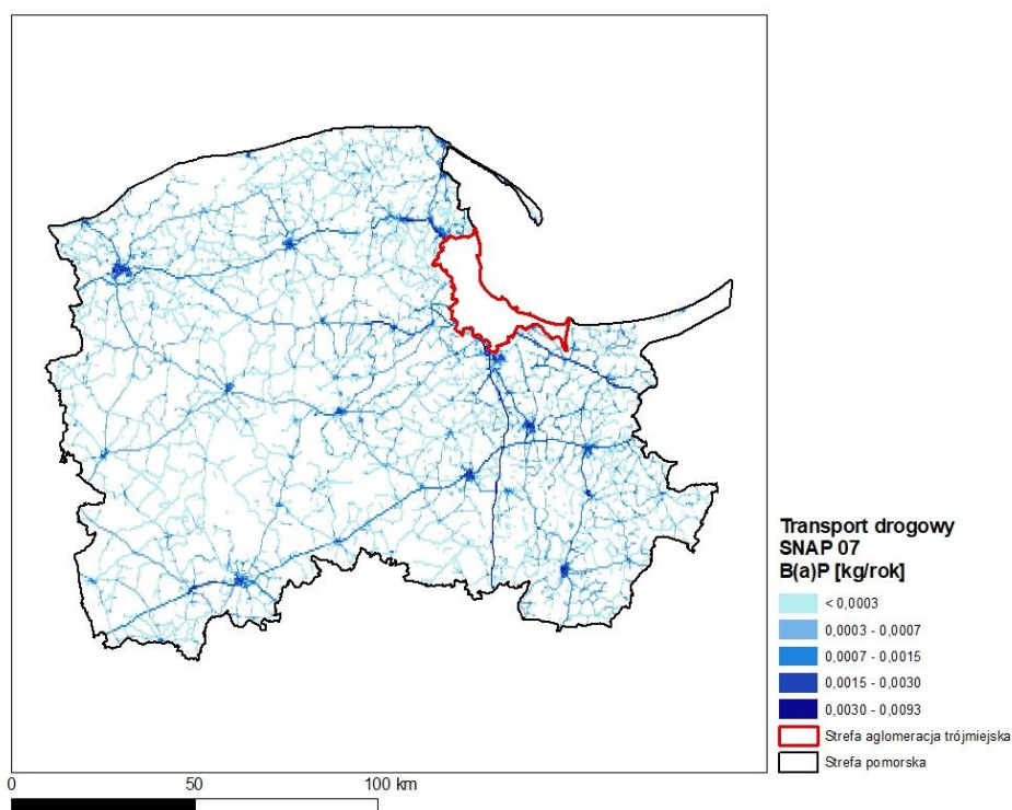
Rysunek 24 Rozmieszczenie oraz ładunki emisji liniowej B(a)P w transporcie drogowym (SNAP 07) w strefie pomorskiej w 2018 r.
